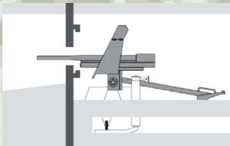
Schemat montażu działka PAK wz. 35/36
